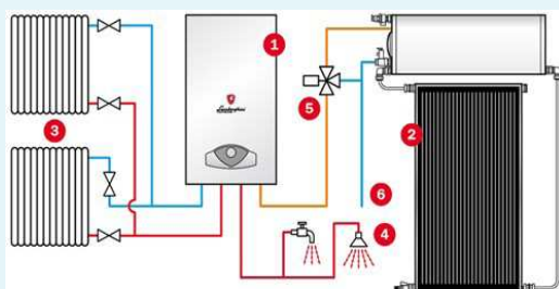
Sistema con n° 1 pannello
